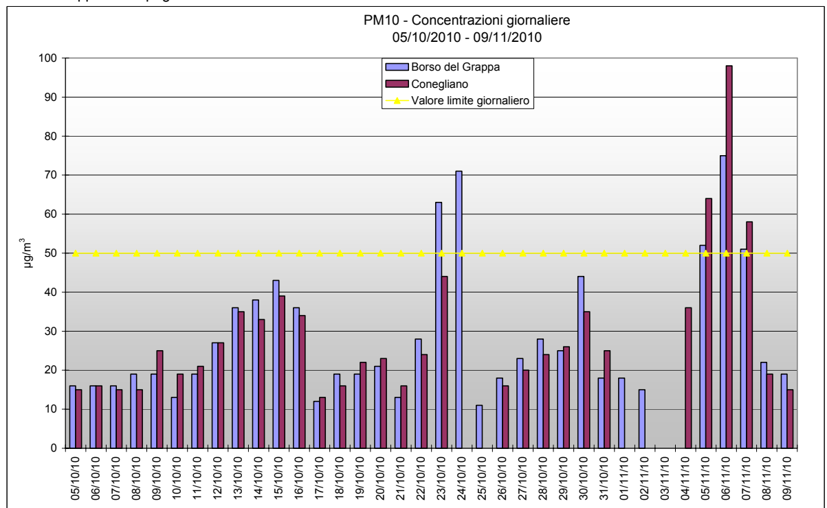
Grafico 2 Valori medi giornalieri di PM10 rilevati presso la stazione fissa di Conegliano ed il campionatore portatile posizionato a Borso del Grappa – campagna invernale
