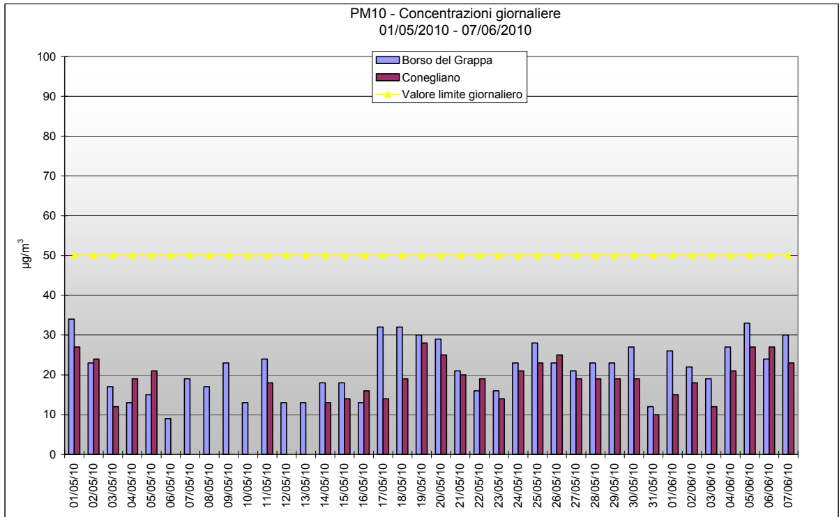
Grafico 1 Valori medi giornalieri di PM10 rilevati presso la stazione fissa di Conegliano ed il campionatore portatile posizionato a Borso del Grappa – campagna estiva.
