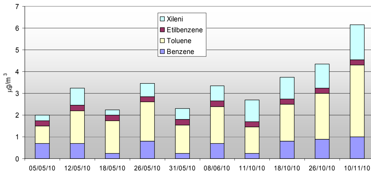
Grafico 3 Valori settimanali di BTEX (Benzene, Toluene, Etilbenzene, Xilene) rilevati a Borso del Grappa.
