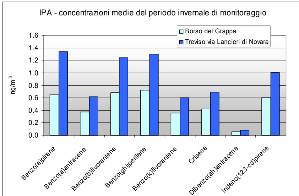
Grafico 4 Confronto tra i valori di IPA determinati su campioni di PM10 prelevati nel sito di monitoraggio e presso la stazione fissa di Treviso durante la campagna invernale.
